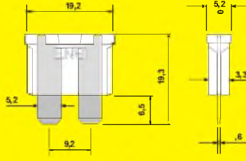
BIÇAK SİĞORTA BLADE FUSE
